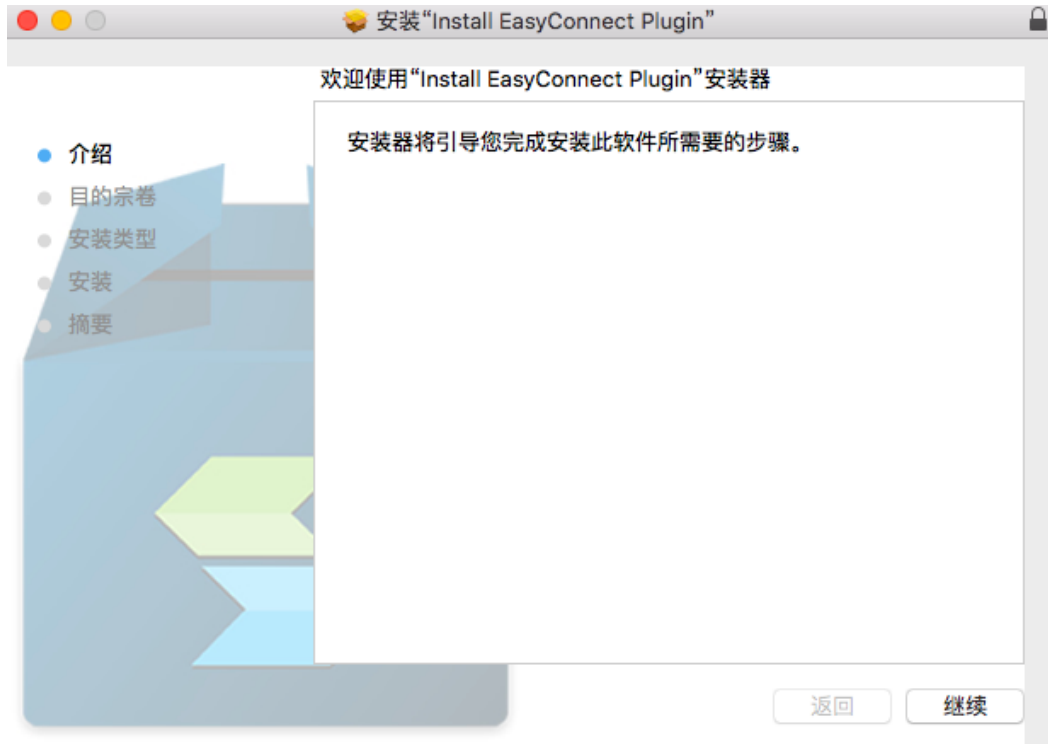
图 10 控件安装器
